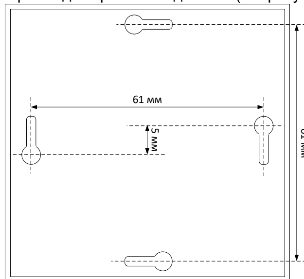
Рисунок 3. Разметка монтажных отверстий
